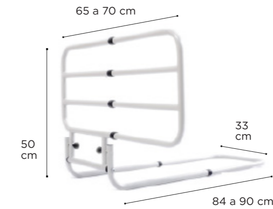
GARCÍA 22601 Asidera y barandilla de cama
